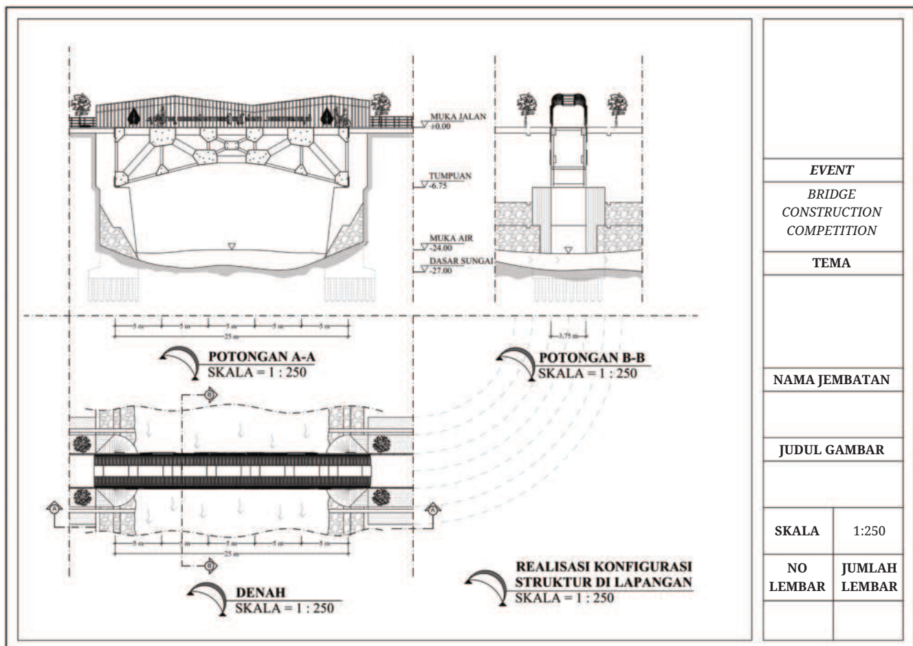
Gambar 5.4 Contoh Gambar Tampak Jembatan
