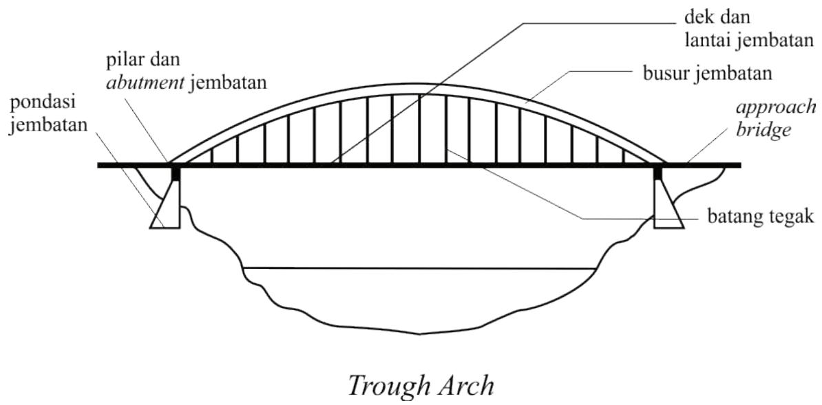
Gambar 5.2 Elemen Jembatan Plengkung
