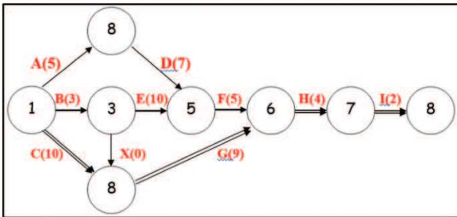
Gambar 6.1 Network Planning dengan Lintasan Kritis
