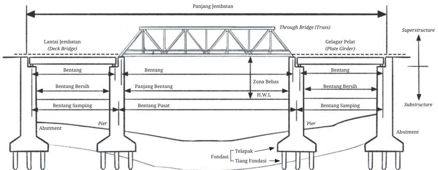
Gambar 5.1 Elemen Jembatan Rangka
