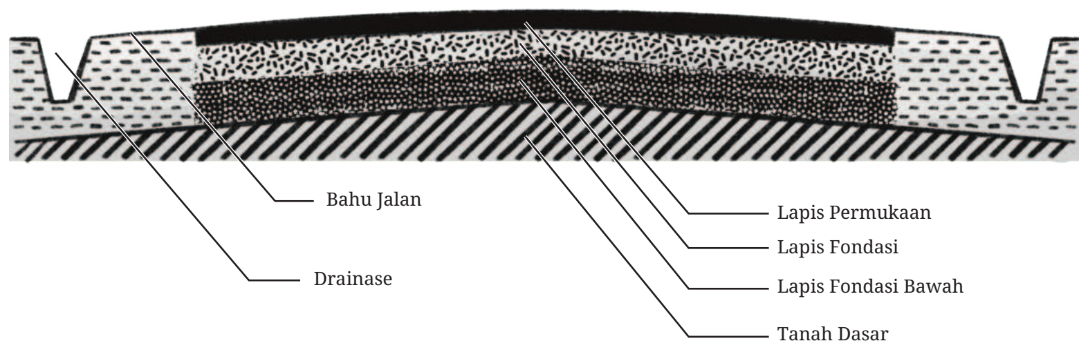
Gambar 3.2 Struktur lapisan fondasi jalan
